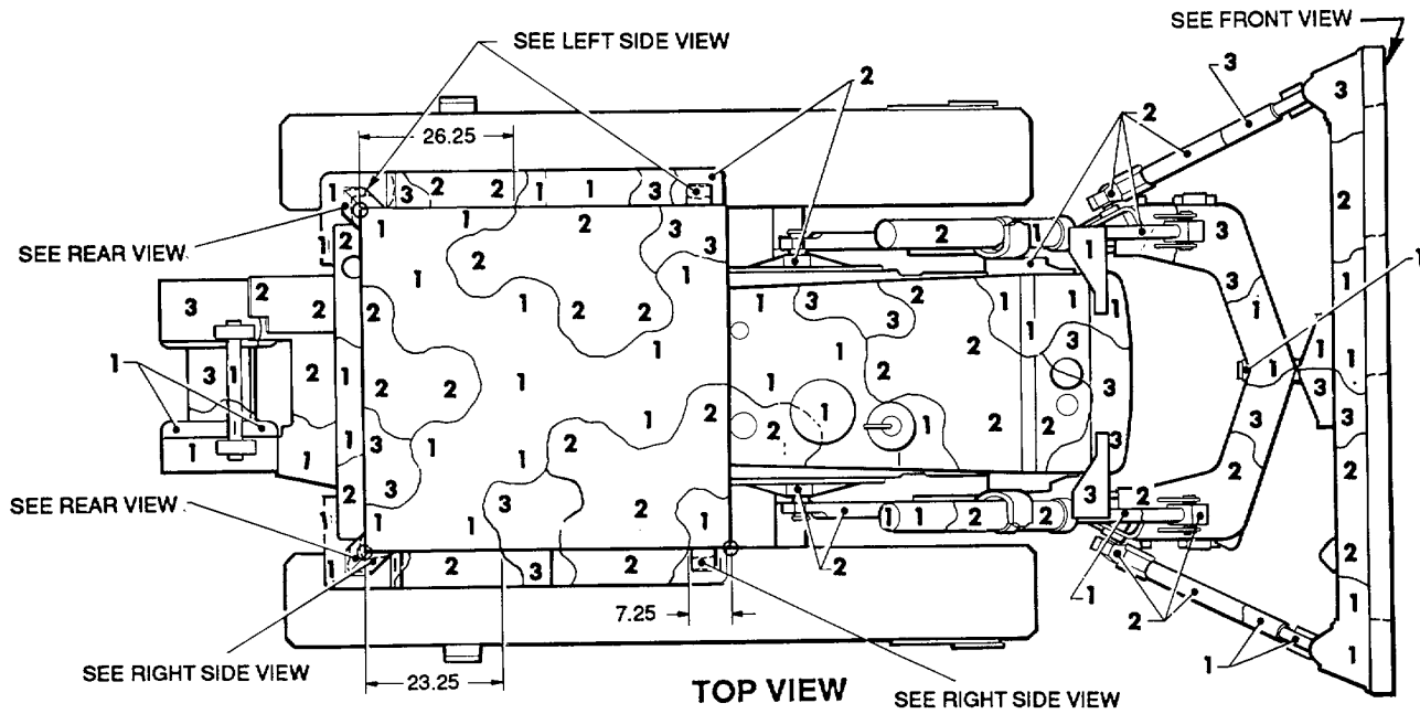
D5BS
