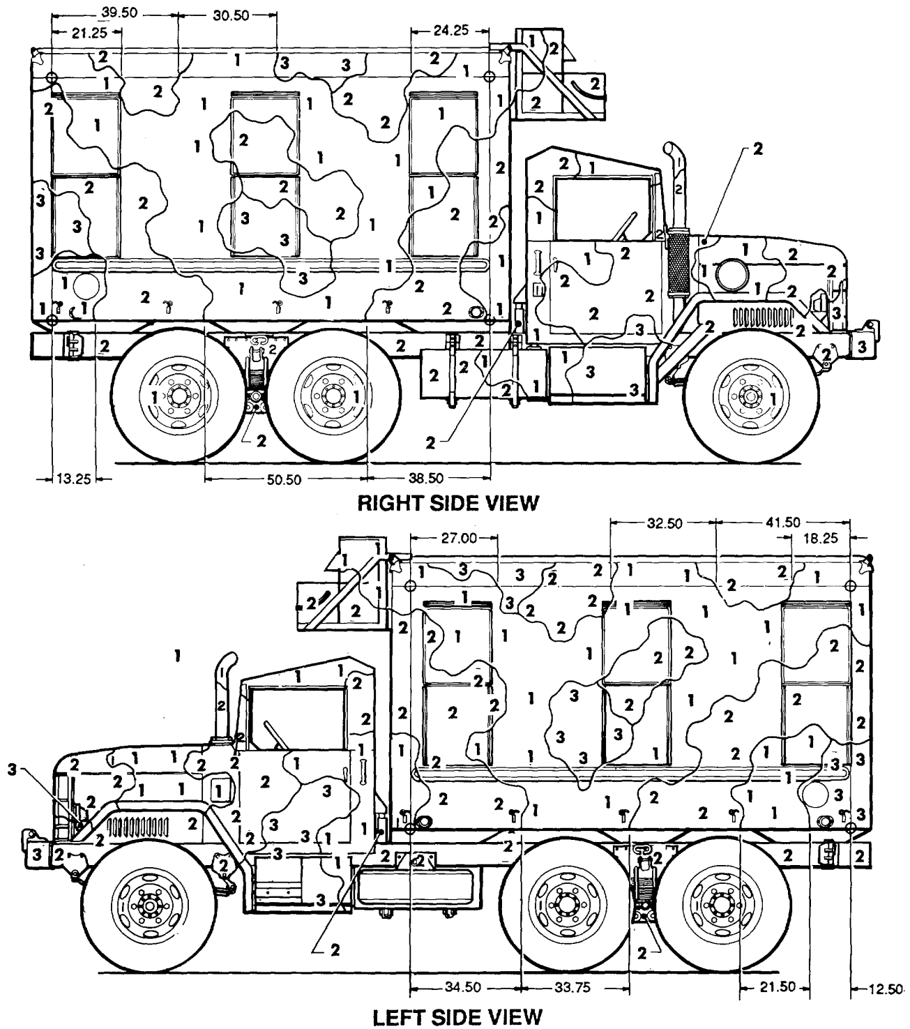
M109A3 M185A3
