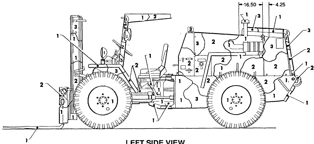
M4K
