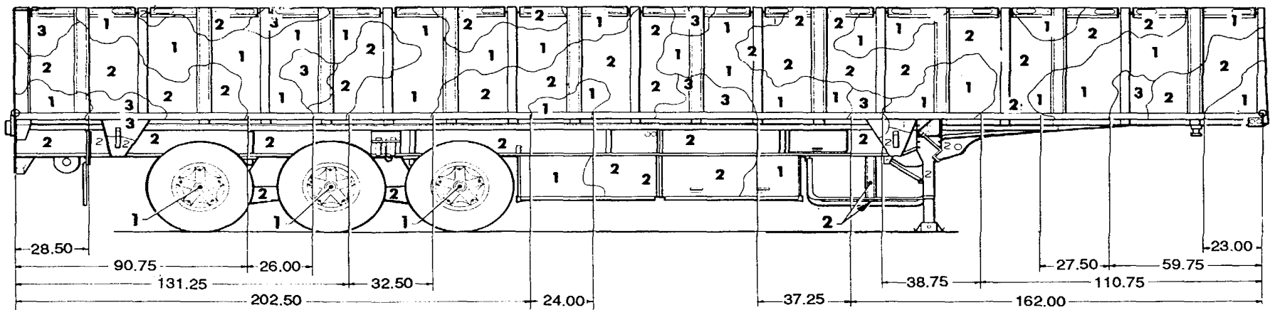
M872A3
